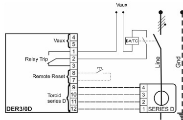
Applicazione con bobina d'apertura (Vaux>48Vca) Application with trip coil (Vaux>48Vac)
