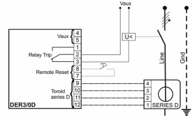
Applicazione con bobina di minima tensione Application with under voltage coil
