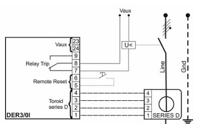
Applicazione con bobina di minima tensione Application with under voltage coil
